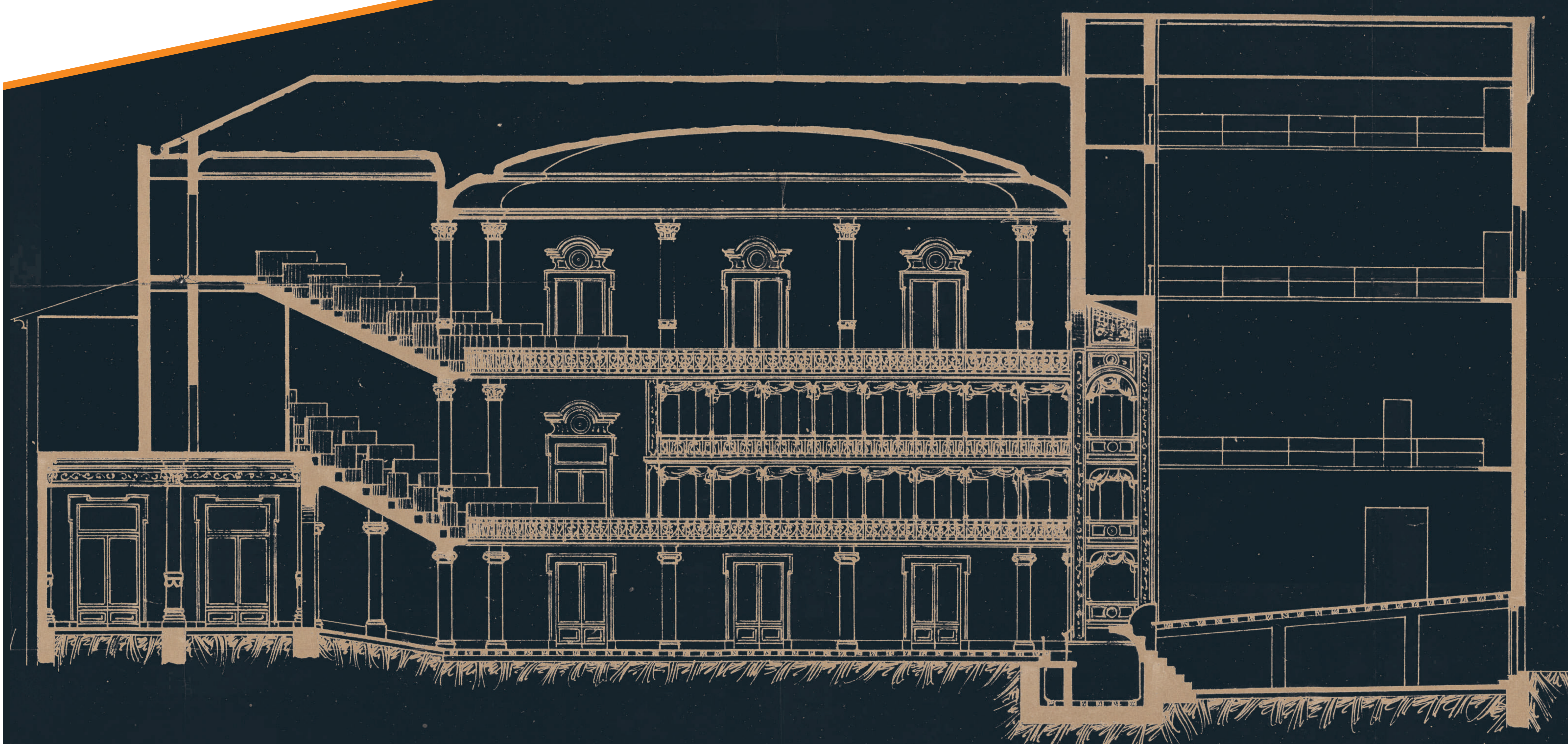
Sez. longitudinale di progetto - Ing. Ido Gazzano
